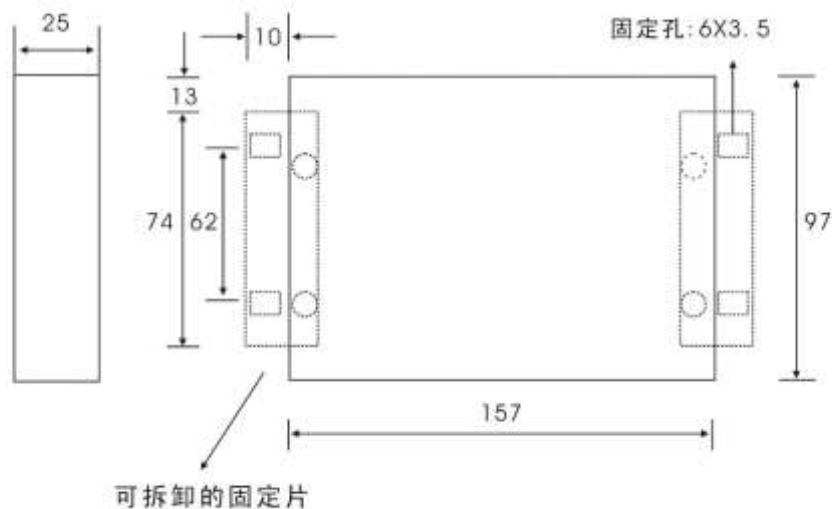
图 2-1 安指示图
