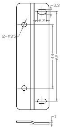
固定片尺寸
