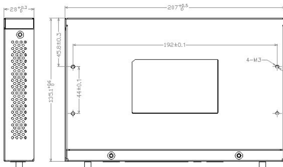
路由器尺寸
