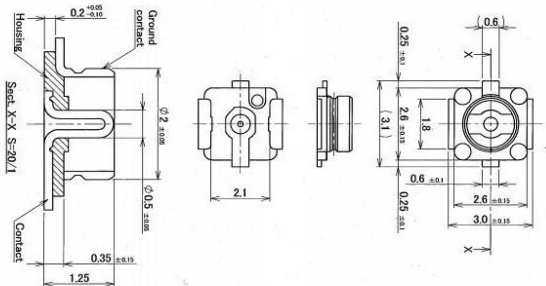
图 2-3 20279-001E-03/IPEX 的结构尺寸
