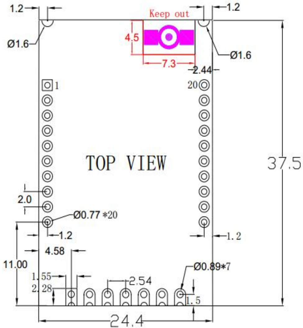
图 6-3 F8L10D-N Outline Package
