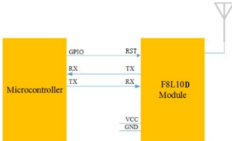
图 3-1 UART 接口连接
