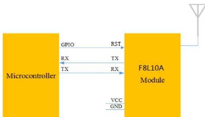
图 3-1 UART 接口连接
