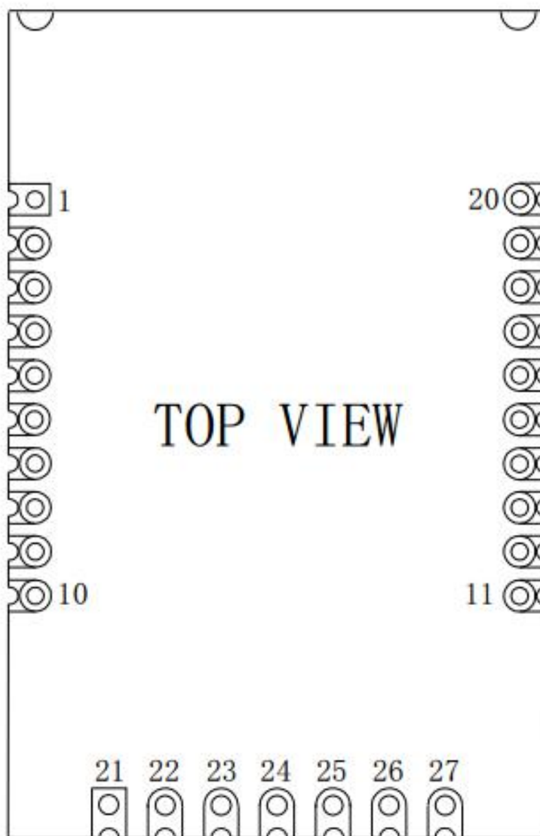
图 2-1 模块引脚图 F8L10A-N 和 F8L10A-E
